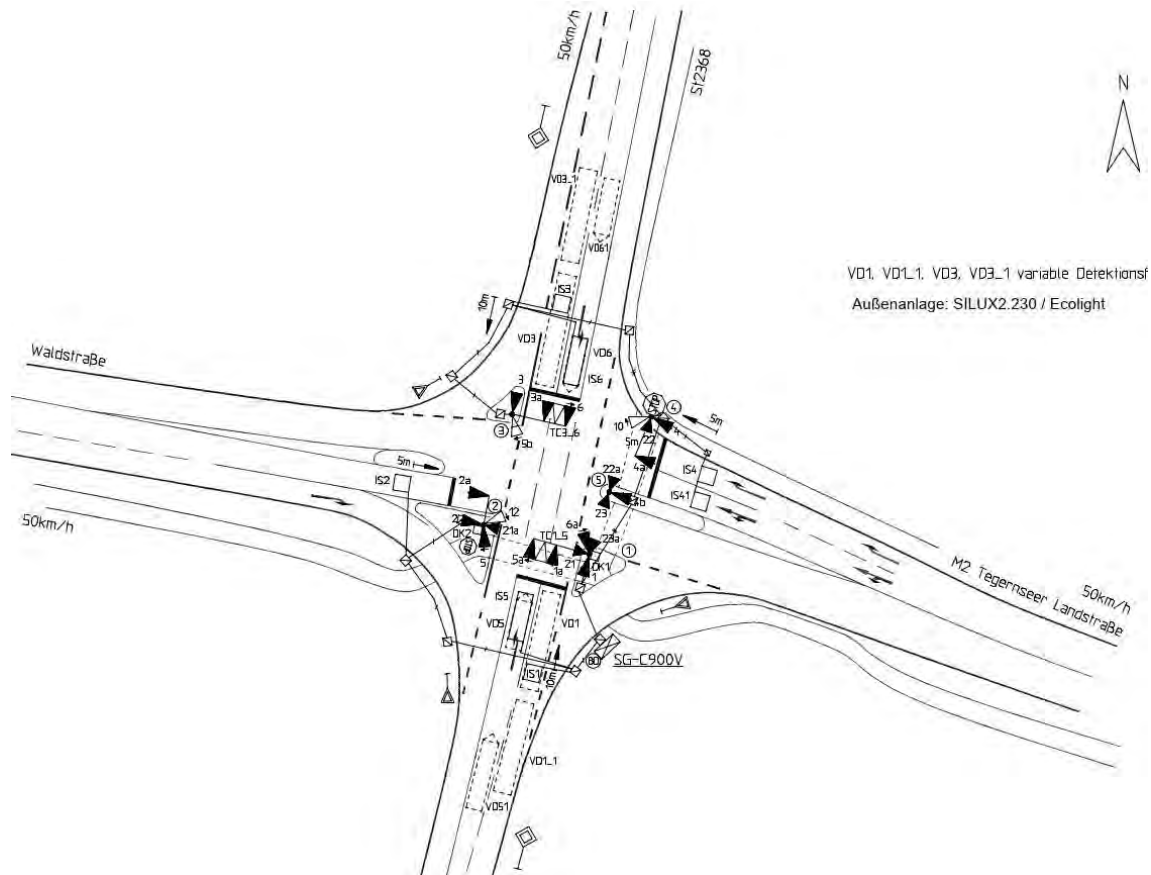
Abbildung 9: Ausschnitt Lageplan Lichtsignalanlage St2368/ M2/ Waldstraße (Quelle: staatliches Bauamt Freising, Siemens Mobility GmbH, 2012/2021)
