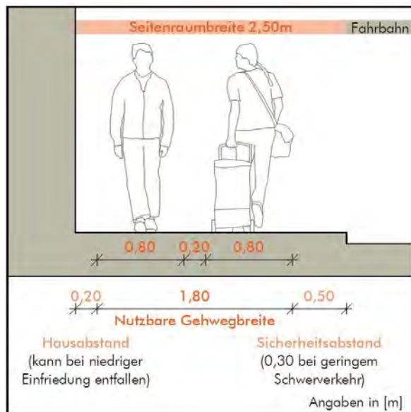
Abbildung 6: Empfehlung für Gehwegbreite (Darstellung PSLV, 2024)
