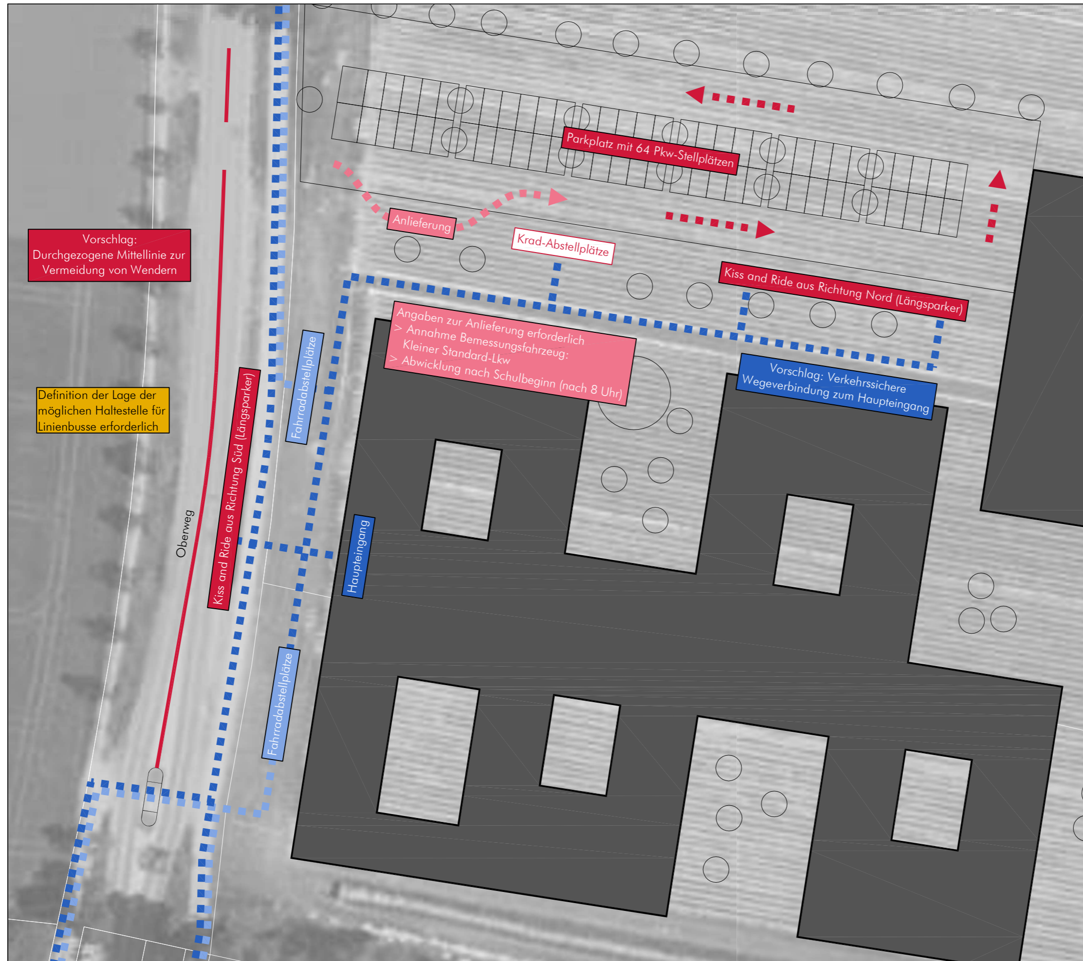
Anlage 2.4 Schemaskizze Erschließungskonzept Übersicht Bildungscampus
